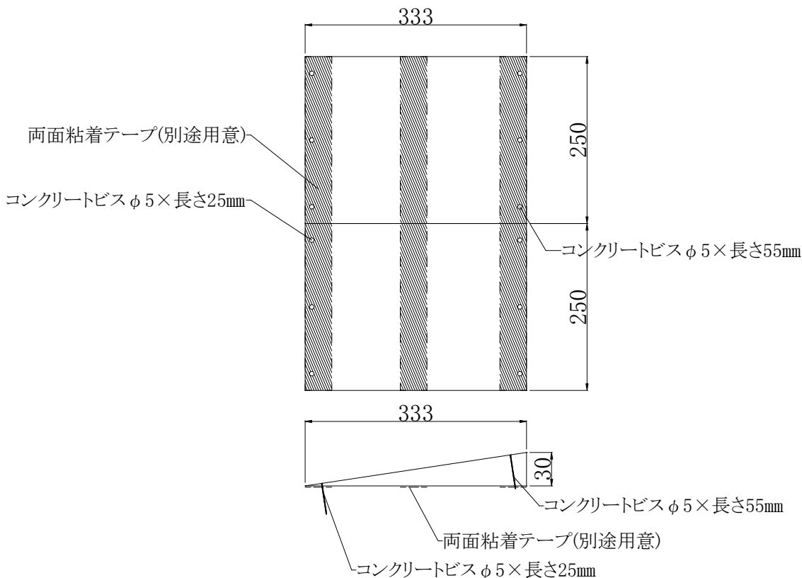
[参考納まり図]
