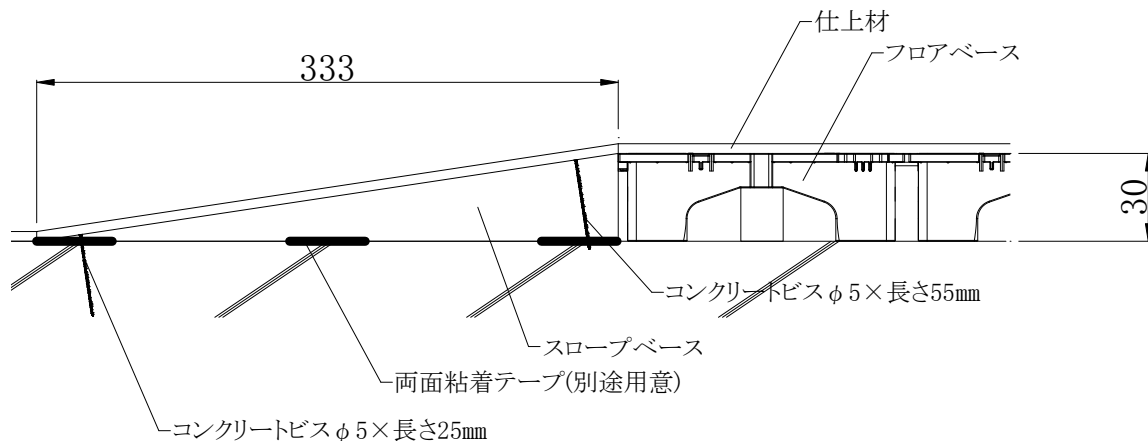
[参考納まり図]
