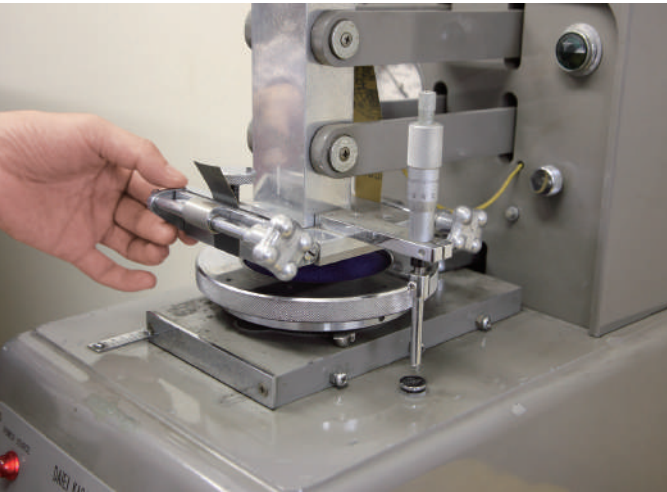
平面摩耗試験機【平面摩耗】 JIS L-1096
