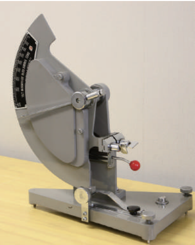
引裂試験機【引裂強度】 JIS L-1096
