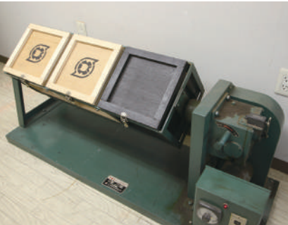
ピリング試験機【毛玉発生確認】 JIS L-1076
