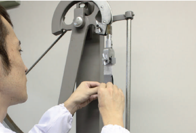
剥離試験機【剥離強度】 JIS K-6772
