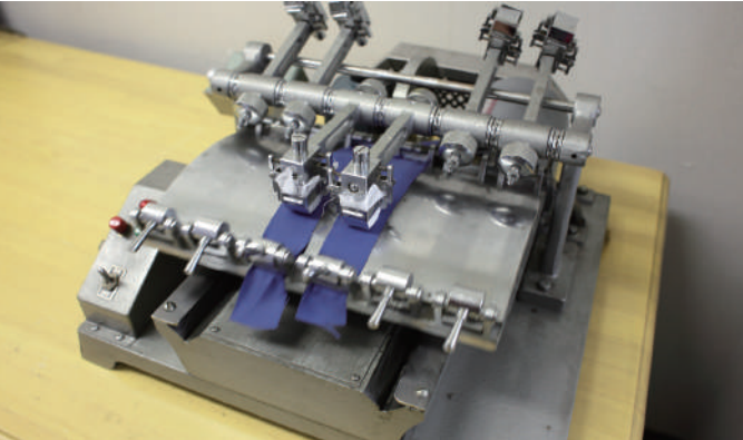
摩擦堅牢度試験機 [摩耗色落ち] JIS L-0849、JIS K-6772
