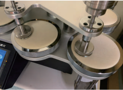
マーチンデール摩耗試験機 (JIS L-1096 摩耗強さE法)
