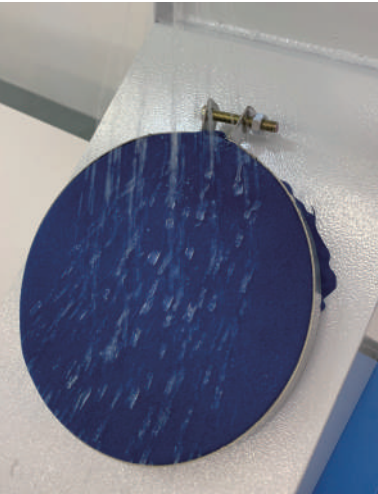
撥水試験機 (JIS L-1092 はっ水度試験 スプレー法)
